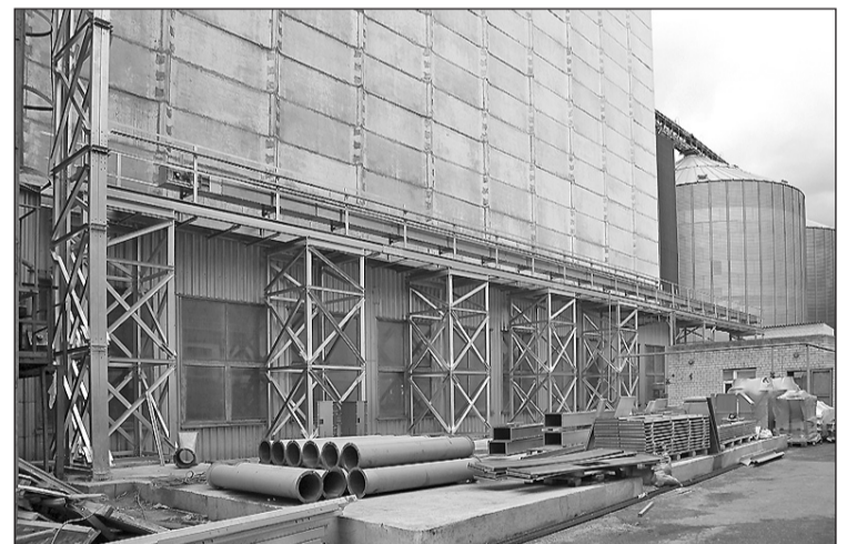
▲ Строительство новой линии транспортировки зерна.
